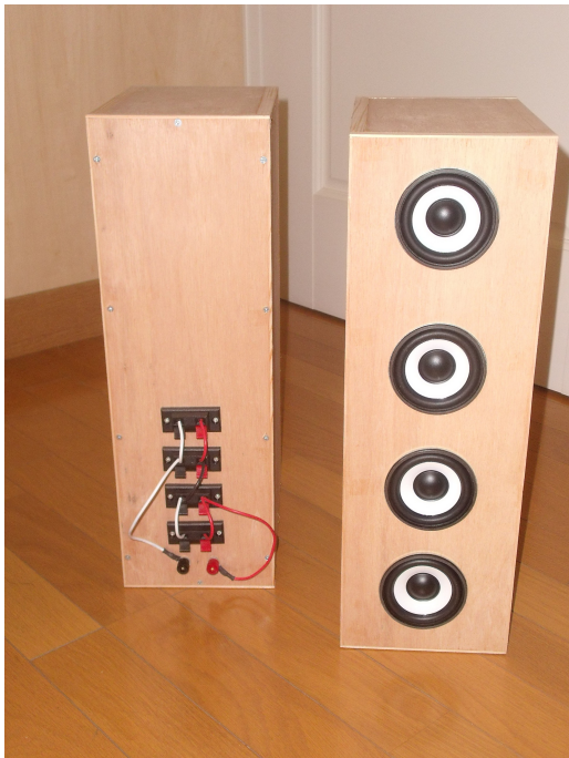
内容積 11.7ℓ 密閉型 鈴木会長が大人買いしたユニット×4
