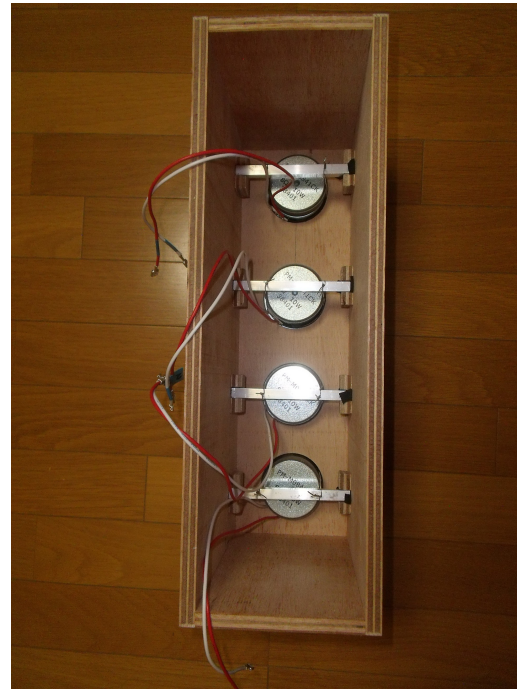
ユニットは背面に渡したアルミ製ブリッジに針金で固定
