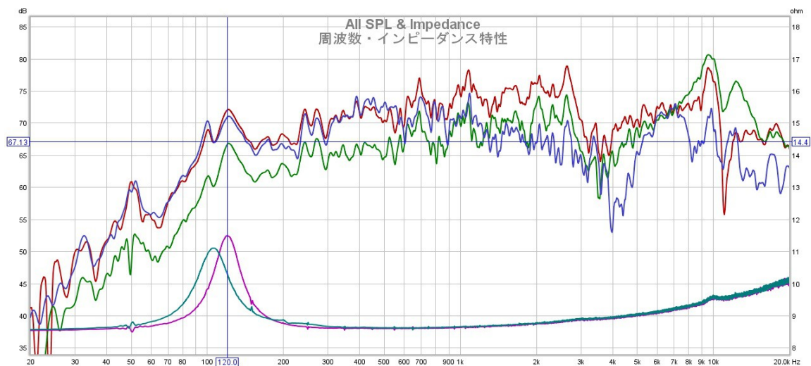
内容積 11.7ℓ 密閉型 鈴木会長が大人買いしたユニット×4
